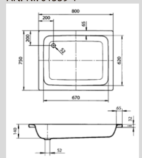
KALDEWEI SANIDUSCH 548-1 Art.-Nr. 01532 5 Art.-Nr. 01549 3 Art.-Nr. 01539 4
