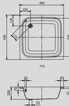
KALDEWEI SANIDUSCH 496 Art.-Nr. 01380 2
