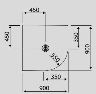
BEFLIESBARE BODENPLATTE Art.-Nr. 81980 0
