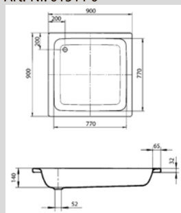
KALDEWEI SANIDUSCH 396-1 Art.-Nr. 01501 1 Art.-Nr. 01524 0 Art.-Nr. 01511 0
