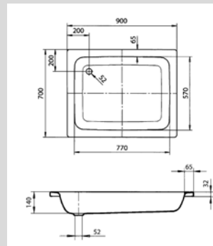
KALDEWEI SANIDUSCH 539-1 Art.-Nr. 01405 2
