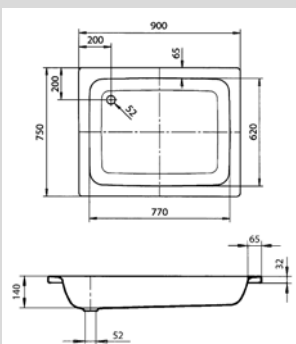
KALDEWEI SANIDUSCH 549-1 Art.-Nr. 01561 5
