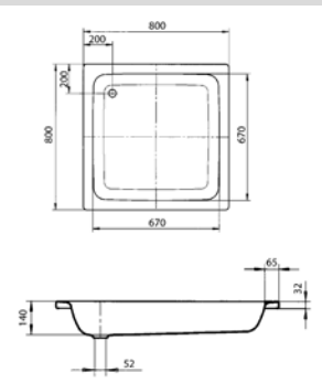
KALDEWEI SANIDUSCH 395-1 Art.-Nr. 01471 7
