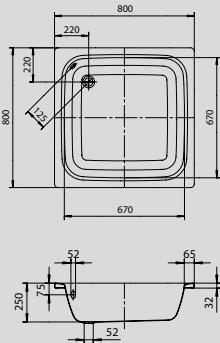
KALDEWEI SANIDUSCH 495-1 Art.-Nr. 01350 5
