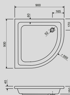
SAMANTHA Art.-Nr. 01683 4 Art.-Nr. 01682 7
