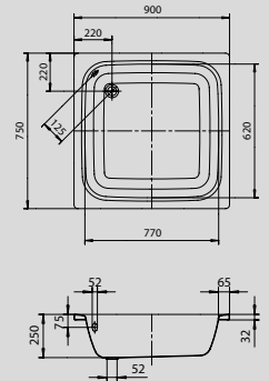
KALDEWEI SANIDUSCH 559-1 Art.-Nr. 01440 3
