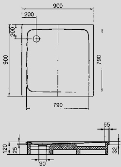
KALDEWEI SUPERPLAN 390-2 Art.-Nr. 01401 4
