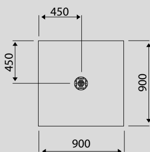
BEFLIESBARE BODENPLATTE Art.-Nr. 81979 4
